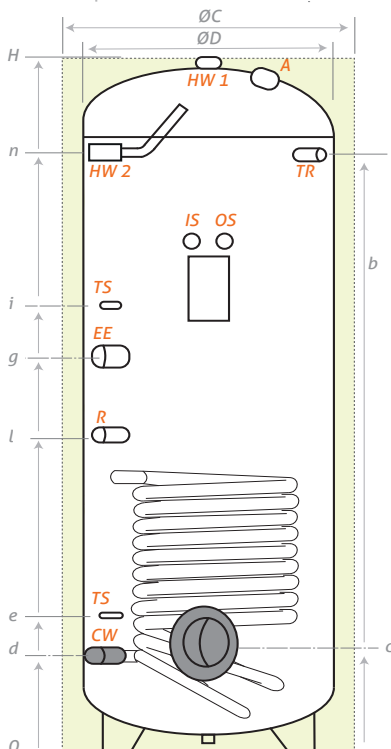
Modèle : 200 litres
