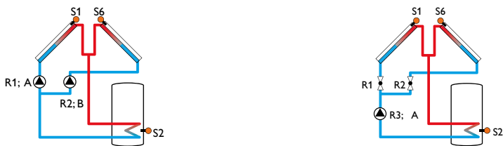
Exemple d'installations avec plusieurs champs de capteurs
